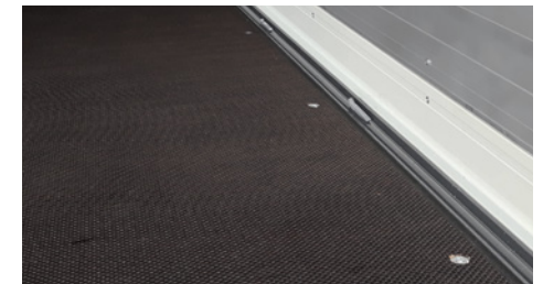
Der Boden des Kofferaufliegers, 30mm wasserdichte, hochfeste Siebdruckplatte. Zulässige Gabelstaplerlast 7,5 t.
