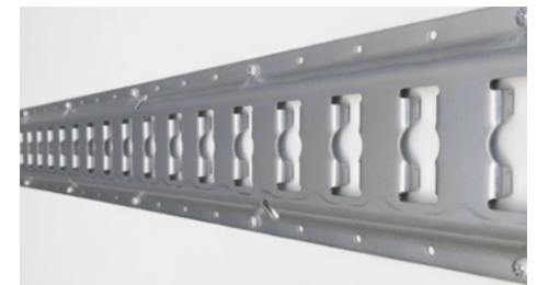
Zurrschienen zur Ladungssicherung, Aluminiumdach.
