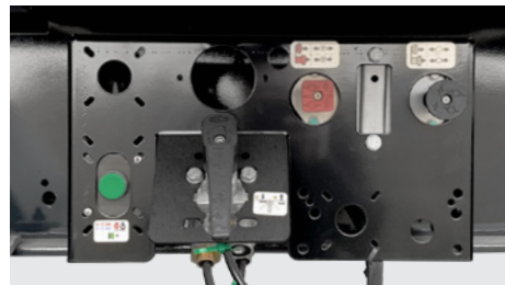
Bedienfeld.
