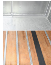
Hintere Ladekante aus Stahl, 700mm.
